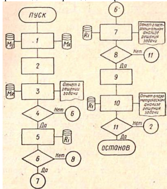
Рис. 1. Укрупненная блок-схема решения задачи оптимизации сельскохозяйственного производства, с использованием пакета прикладных программ [LPS] и базы данных построенной на основании унифицированных блоков экономико-математической модели:
