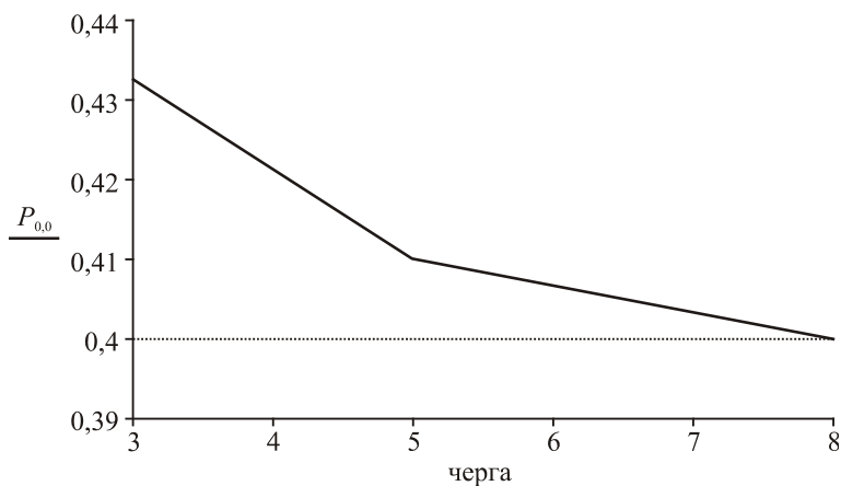
Рис. 2. Динаміка зміни ймовірності простою підприємства, залежно від розміру черги
