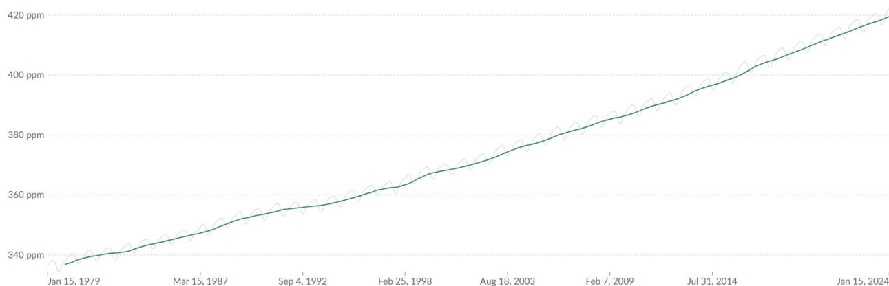
Рисунок 2.1 Глобальна концентрація CO 2 в атмосфері [23]
