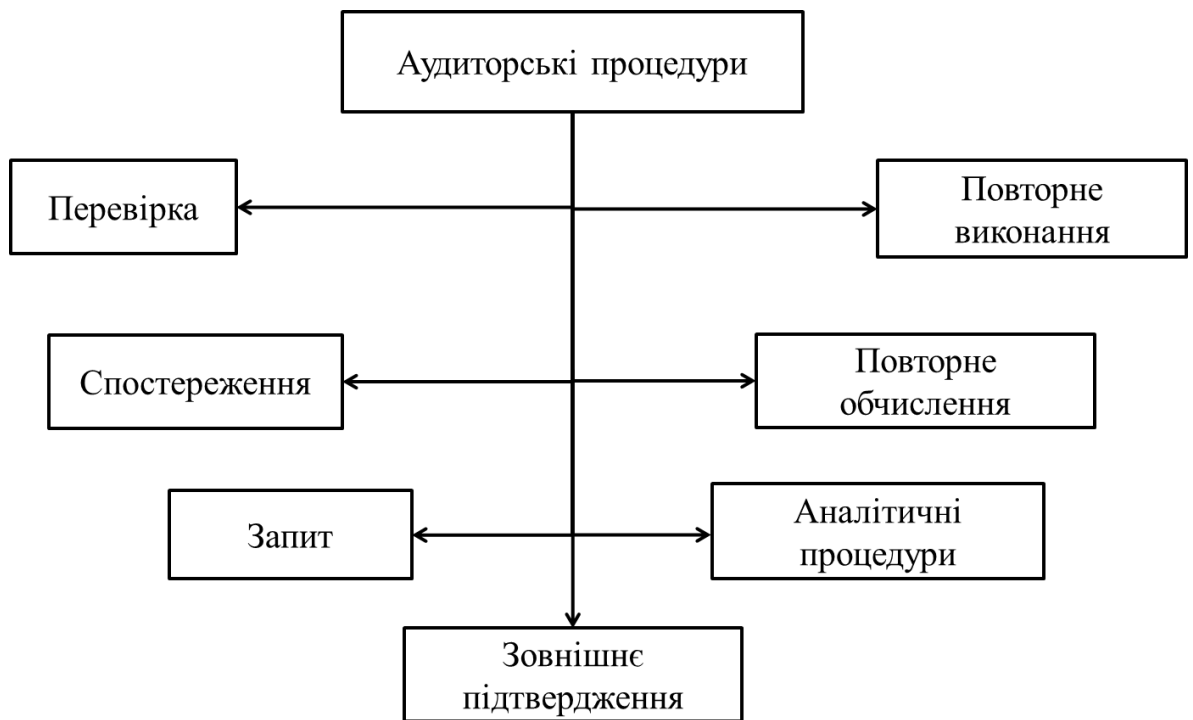
Рисунок 3.11 – Процедури аудиту
